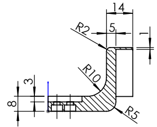
剖面 A-A
